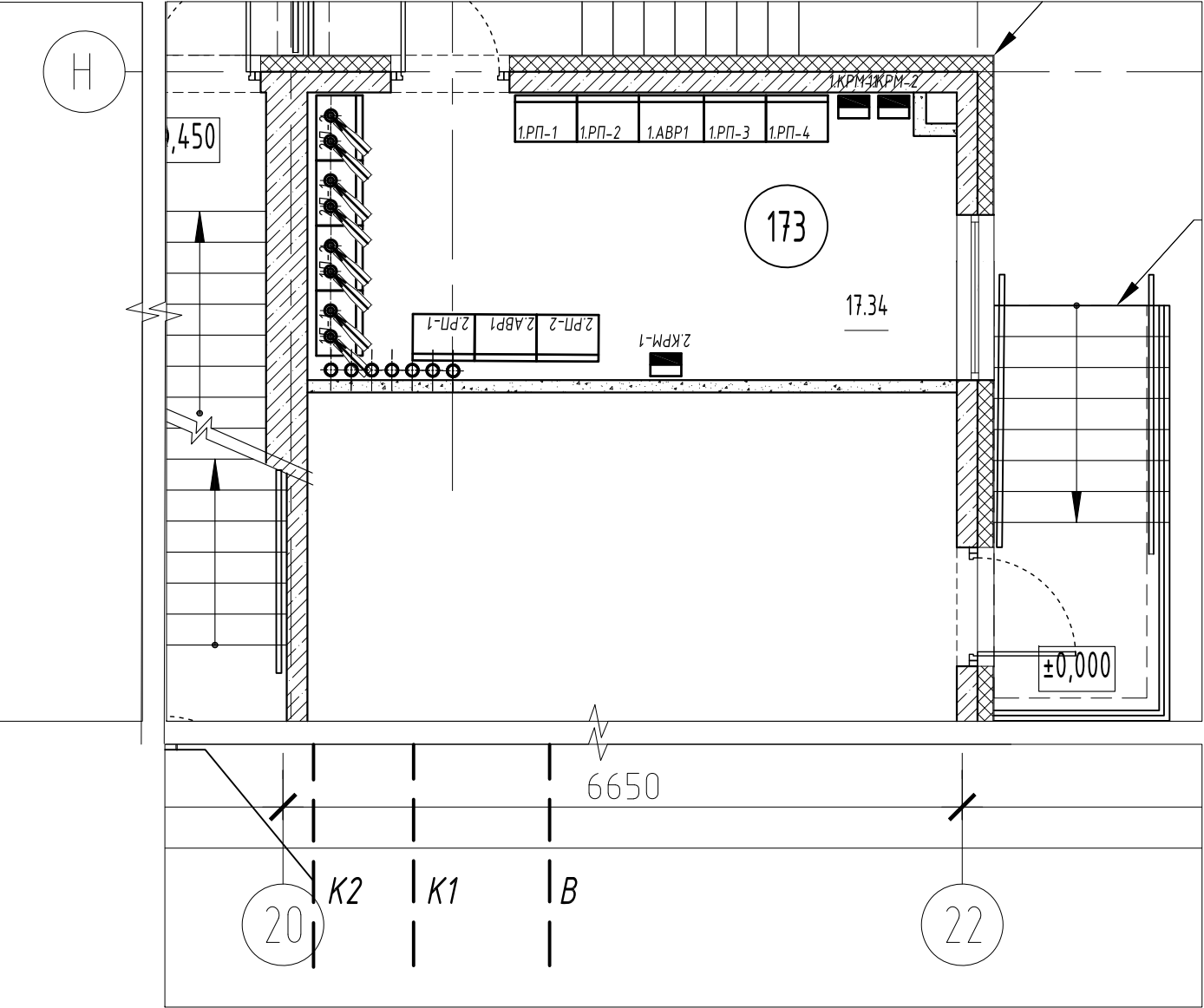
План расположения силовых щитов ВРУ
